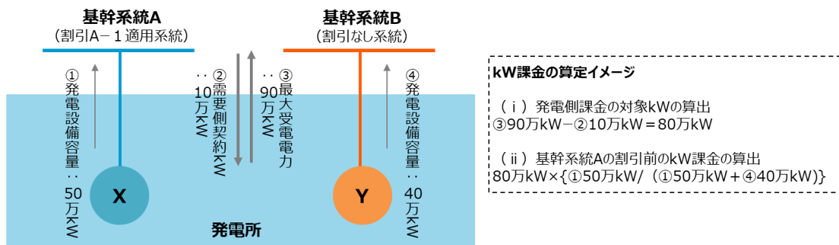
【図表 21】異なる基幹系統等に連系している場合の割引適用イメージ
